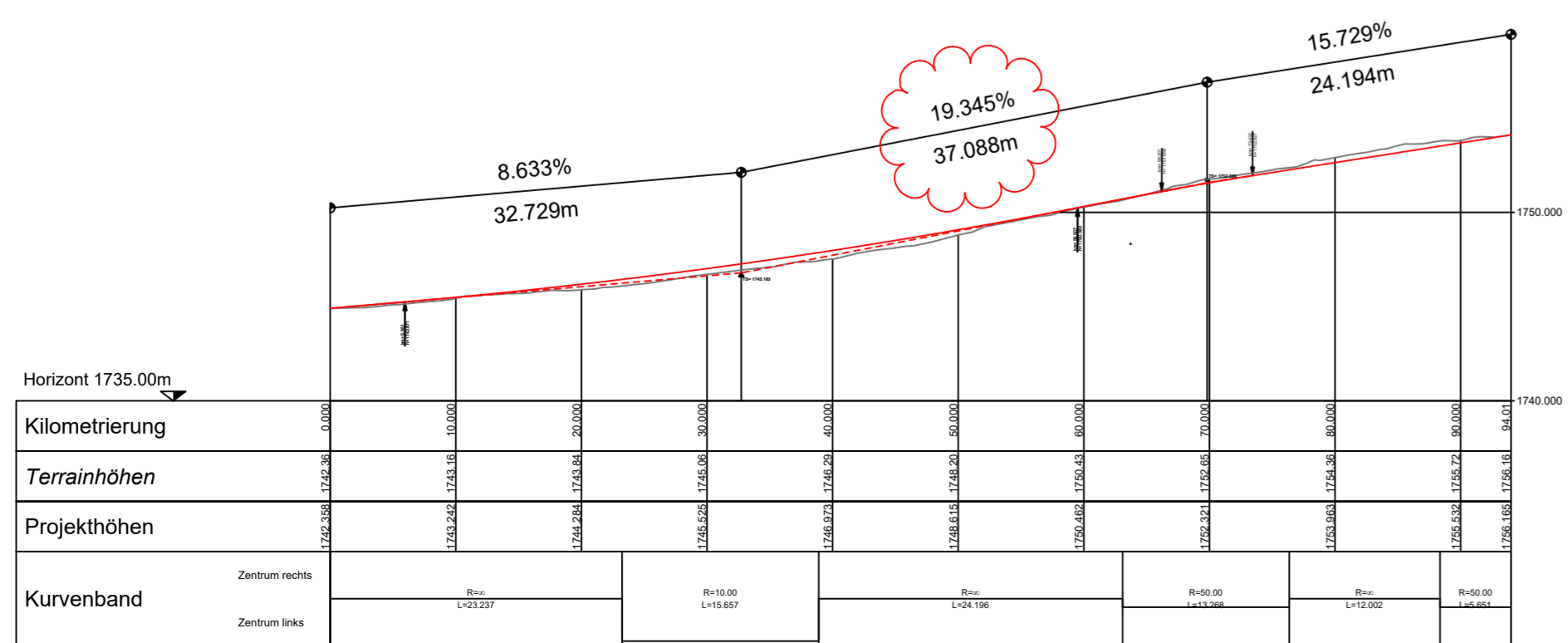
Längenprofil Fussweg Breite 2.50 m
