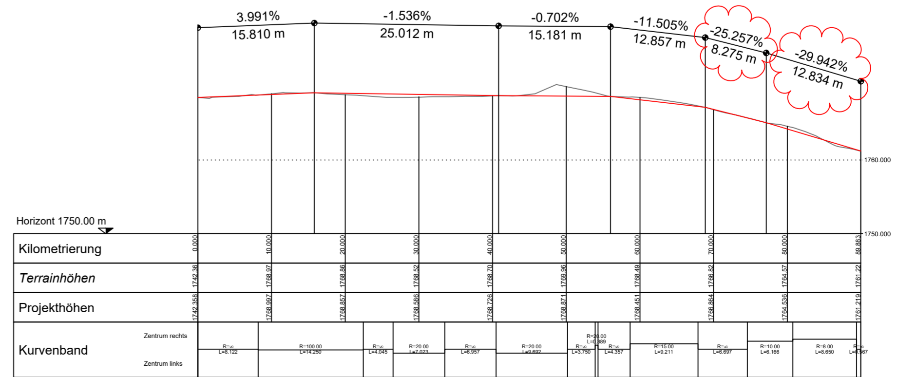
Längenprofil Fussweg Breite 1.50 m
