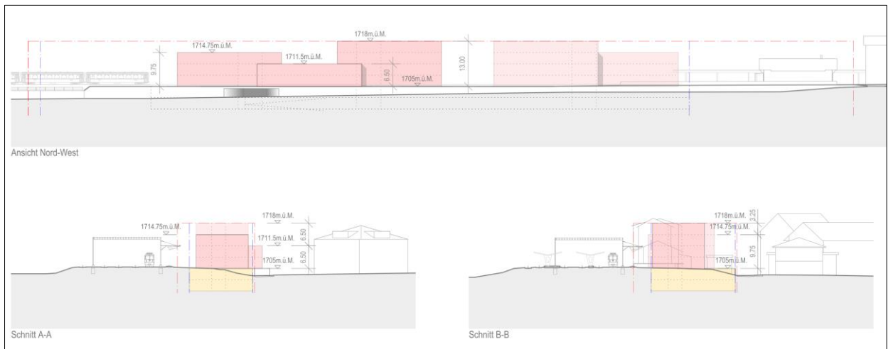
Ansicht Nord-West und Schnitte, Machbarkeitsstudie Variante 9 (nicht massstäblich), Liesch Ott Architekten
