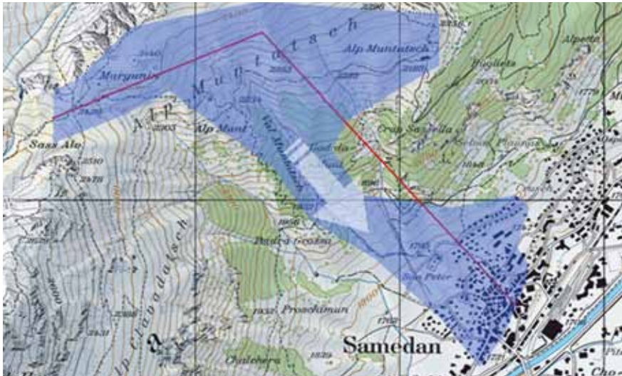
Abb.: Profil des konzeptionellen Grundwassermodells und Fließpfad
